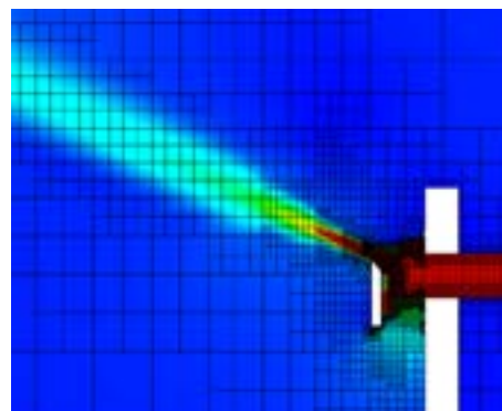
Simuleringsbild som visar hur avluften transporteras från fasaden genom en uppåtriktad luftstråle.
