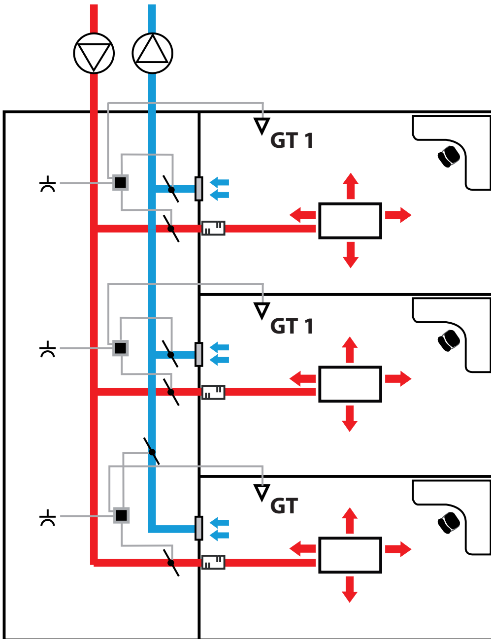
System ABC-VAV Kontroll (exempel)
