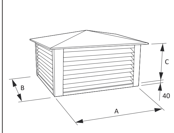
Exempel takgenomföring TGTH 2 anslutningar.
