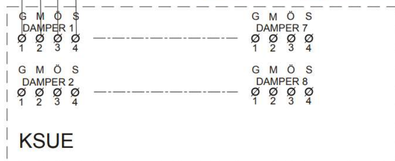
Anslutning av ett spjäll utan KBOX.
