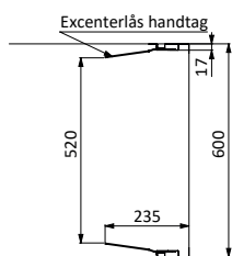
Skissen ovan visar innermått vid användning av ABC-EXL excenterlås.
